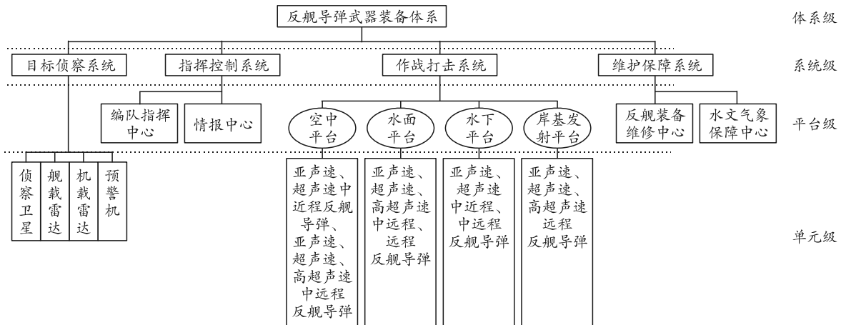
图 4 反舰导弹体系层级结构 OCV-6a 模型
